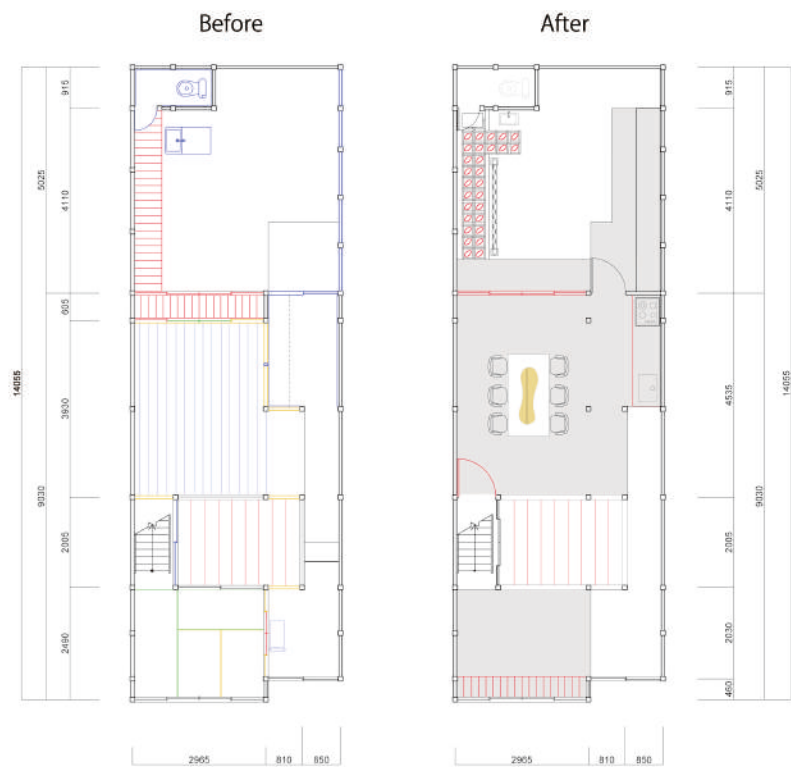
平面図 1/100
