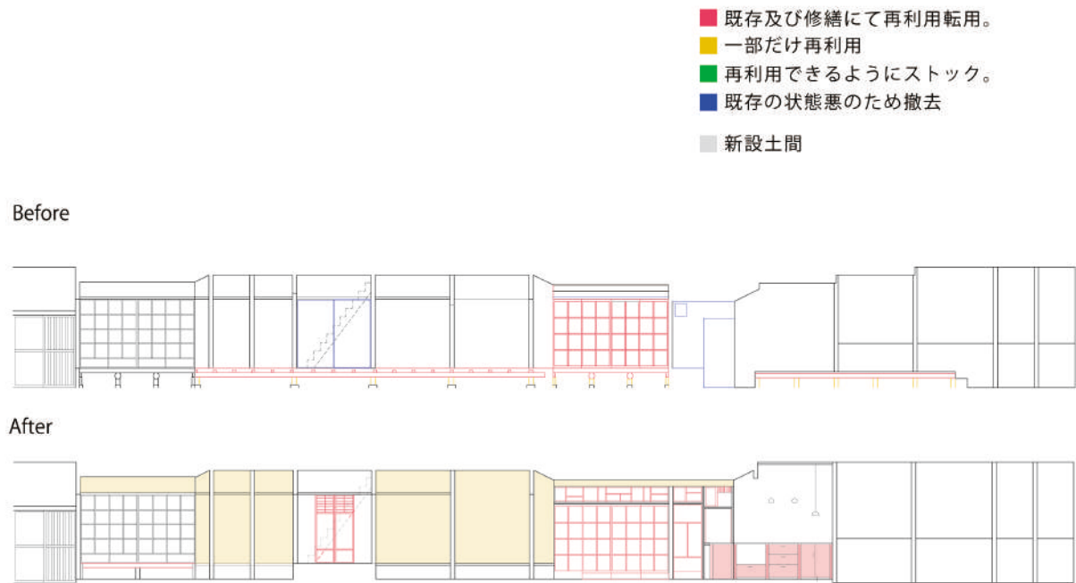
展開図 1/100
